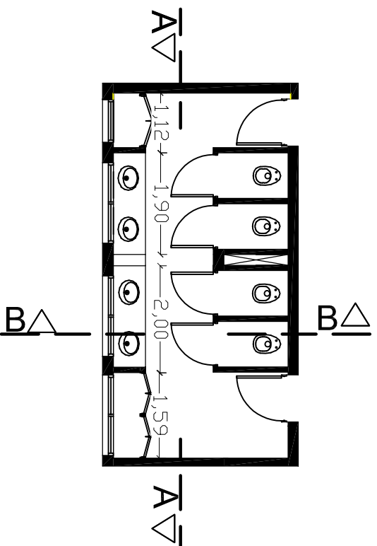
Planta remodelada
